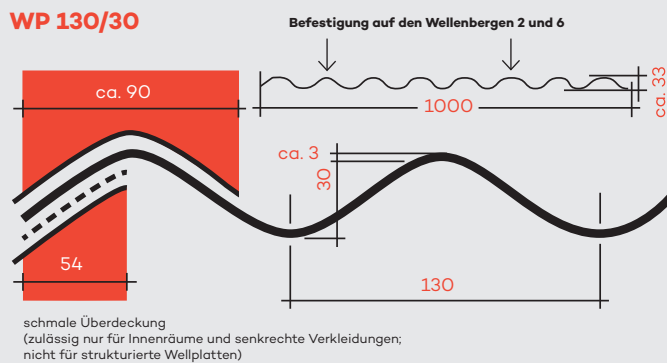
Querschnitt der PLEXIGLAS® Resist WP 130/30 (Maße in mm)
